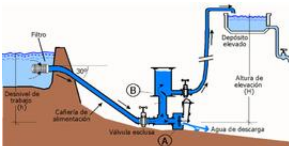
Esquema demostratiu de la tècnica de l'ariet hidràulic. Font: Viquipèdia.
